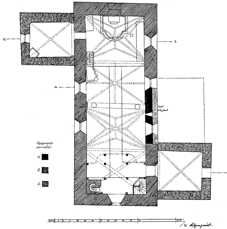
Plan av kyrkan mot öster. Uppmätt av A Liljenquist och D Blomquist 1912. Sveriges kyrkor.
