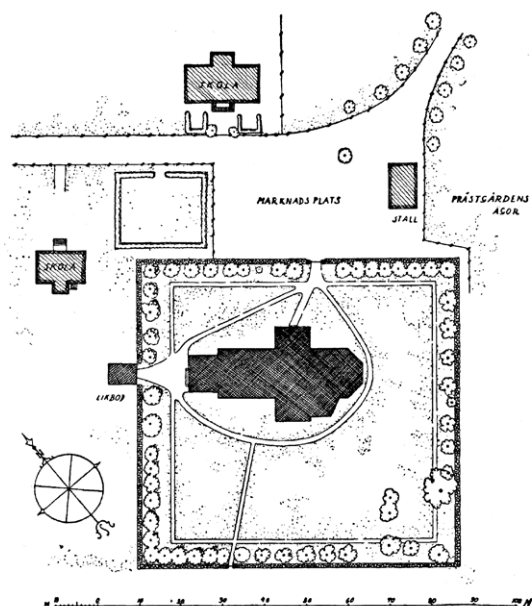
Plan av Vallentuna kyrka mot norr. Uppmätning från 1921, kompletterad 1948. Efter Sveriges kyrkor.
