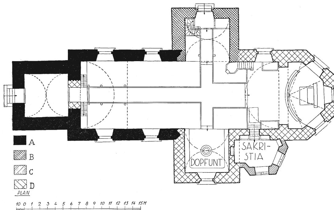
Plan av Vallentuna kyrka mot norr. Uppmätning från 1921, kompletterad 1948. Efter Sveriges kyrkor.
