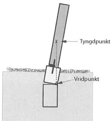
Figur 14. Otillräcklig förankring i undersockel eller gjutning, fall 2.
