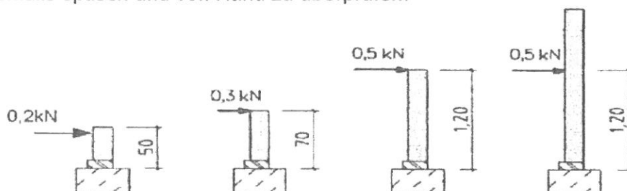
Bild 1: Horizontalbelastung
