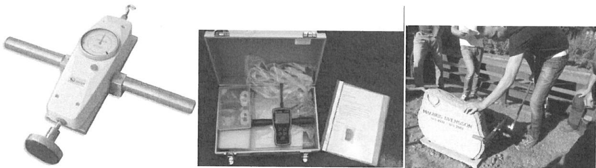
Figur 19. Tre gravstensinstrument. Till vänster FA-500 G från Elastocon AB, Brämhult, i mitten Sauturs instrument komplett i väska och med handledning på svenska, från SweTest, Saltsjö-Boo, Båda med tydlig display, tryckplatta och dragkrok och till höger det av Orax speciellt framtagna instrumentet för prövning av gravstenssäkerhet.
