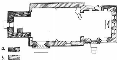
Grundplan över Ekeby kyrkas äldre byggnadsdelar med de olika bygpperioderna markerade (a. 1100-talets slut, b. 1200-talets slut).
