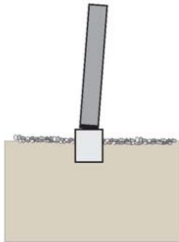
Figur 2. Stenen ser ut att stå stadigt men dubben är otillräcklig eller saknas helt, hålls fast enbart av tjärpapp eller lim
