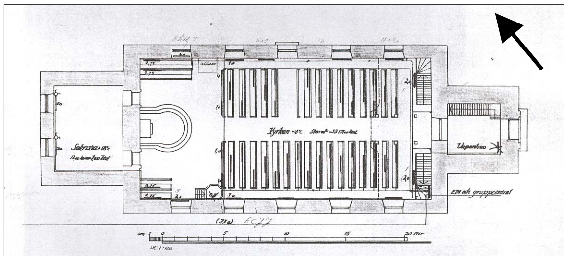
Plan över kyrkan, uppritad i samband med installation av elektrisk värme. Plan av Edw. W Magnusson, 1946.
