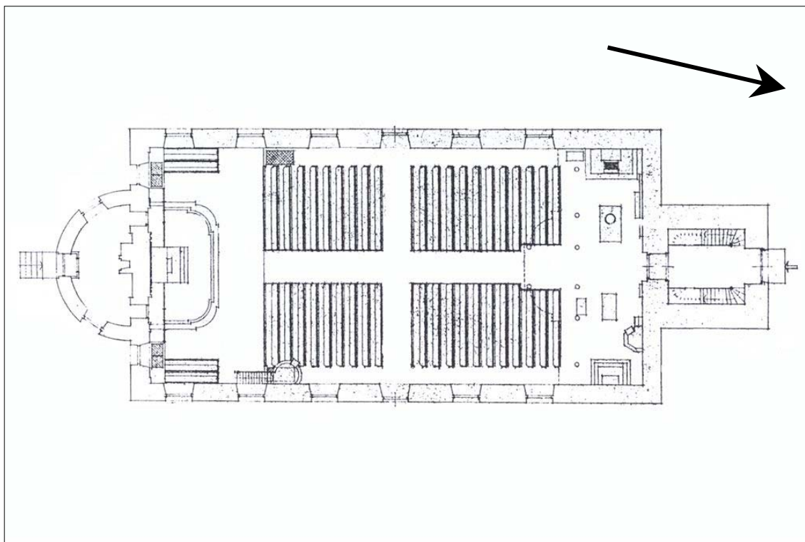
Flisby kyrka. Plan upprättad i samband med installation av bänkvärme 1960 av Johannes Dahls arkitektfirma, Tranås. Kopia av ritning i Jönköpings länsstyrelses arkiv.
