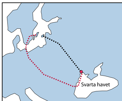
Vägen från Dagö till Ukraina 1781 (svart linje) och vägen till Sverige 1929 (röd linje).
