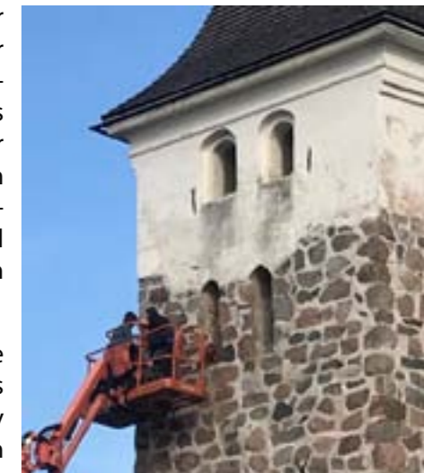
Inspektion av Balingsta kyrkas torn. Foto: Johan Lautmann
