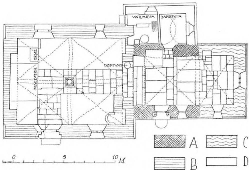
Plan. Byggnadsperiod A: 1200-talets förra hälft, – B: 1200-talets andra hälft, – C: 1300-talets mitt och – D: 1860. Sakristians innervägg ligger idag väster om fönsteröppningen mot norr. Uppmätning omkring 1920. Efter Sveriges Kyrkor, Gotland I:5, volym 35.
