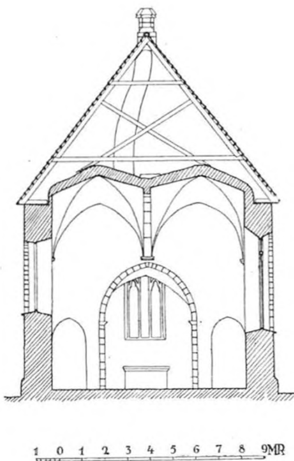
Tvärsektion av långhuset mot öster. Uppmätning omkring 1920. Efter Sveriges Kyrkor, Gotland I:5, volym 35.
