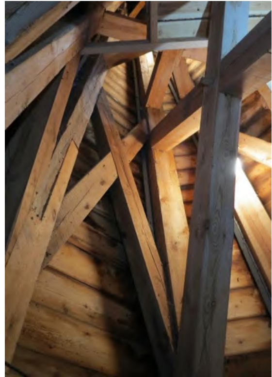
Takryttarens konstruktion av tornhuven ovanför klockvåningen. Foto JL 2019.
