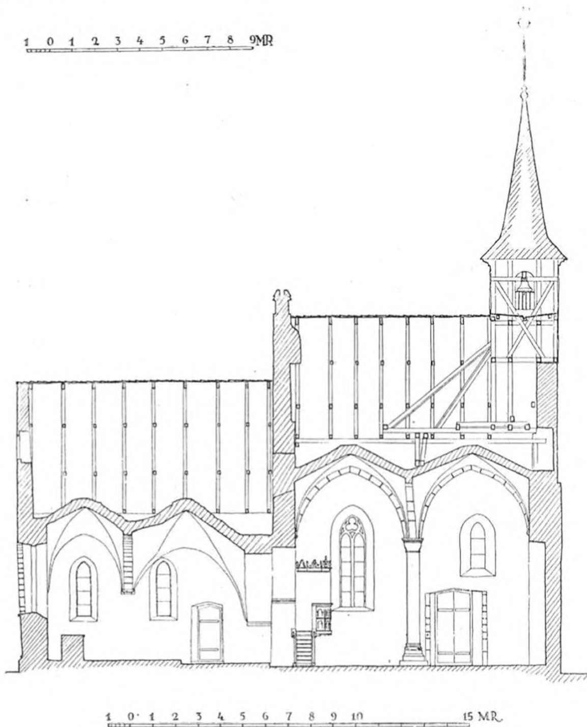
Längdsektion mot söder. Det två linjerna genom långhusets östgavel i nivå med valven markerar läget för passagen mellan kor- och långhusvind, placerad i svickeln mellan sidoskeppens valv, medan sektionens snitt ligger mitt i norra sidoskeppet. Uppmätning omkring 1920. Efter Sveriges Kyrkor, Gotland I:5, volym 35
