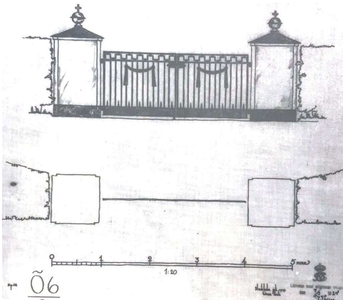
1923. Ritning - Förslag till ny grind. Kyrkogårdens södra gindparti (ATA).
