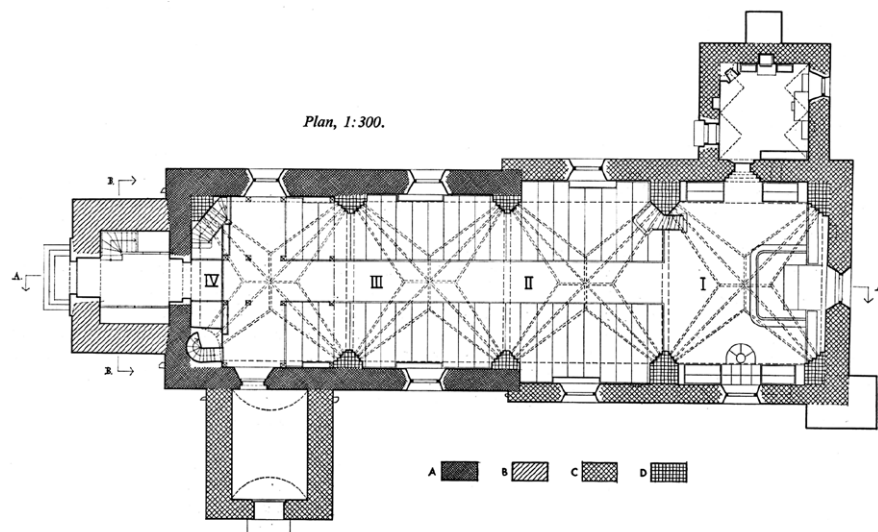
Plan av Botkyrka kyrka. Uppmätning Å Seberg och J E Österberg 1930. Ur Sveriges kyrkor.
