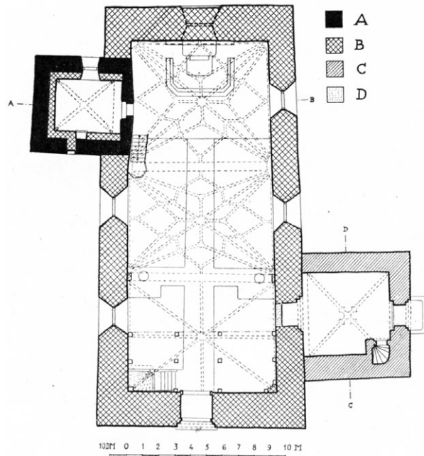
Plan över Kårsta kyrka mot öster. Uppmätning av A Liljenquist 1912, reviderad av A Tuulse 1950. Efter Sveriges Kyrkor.
