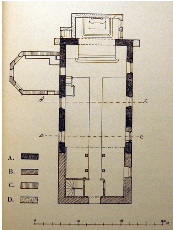
Plan, uppmätning av S Brandel 1916, ur Sveriges kyrkor, 1918.
