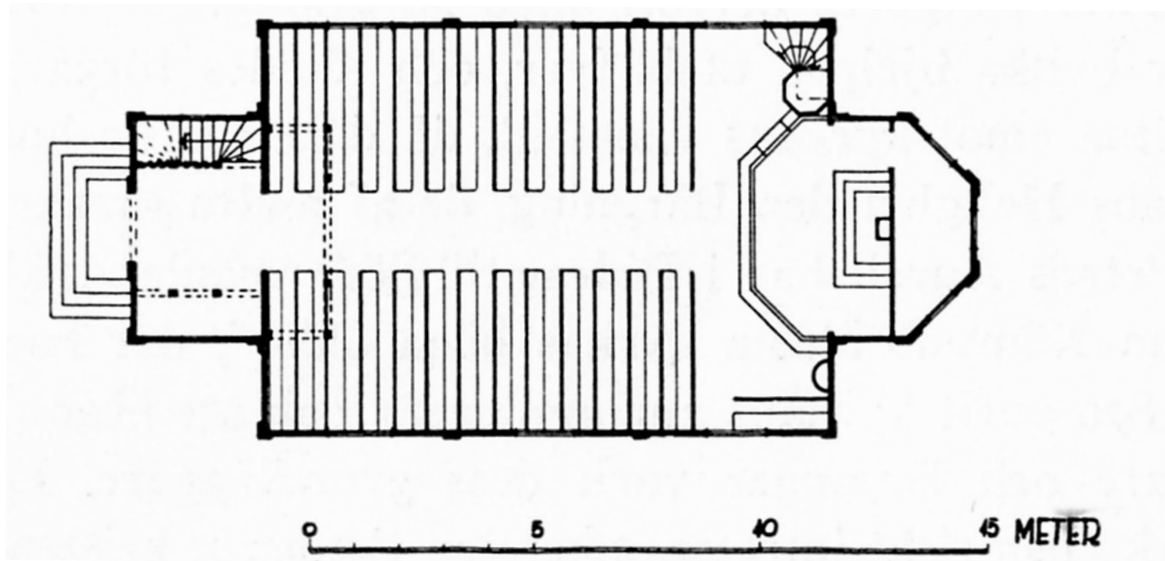
Plan över Nämdö kyrka mot norr. Ur Sörmländska kyrkor 1948.
