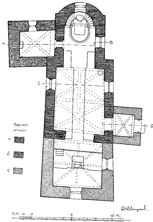
Plan över kyrkan ur Svanberg, Jan, Orkesta kyrka, Upplands kyrkor, Del IX, Uppsala 1967.
