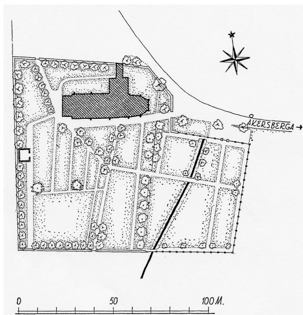
Kyrkogårdsplan. Uppmätning av J Söderberg 1948. Sveriges kyrkor.
