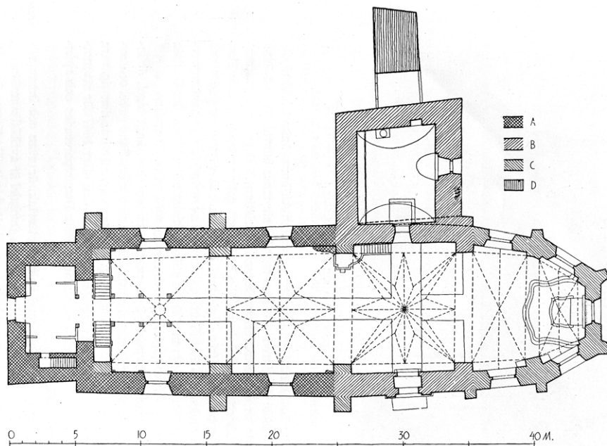
Plan av kyrkan mot norr. Uppmätning av B Wijkmark 1913, reviderad av P O Westlund 1945.
