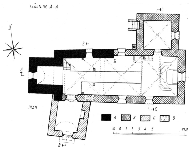
Plan över kyrkan ur Tuulse, Armin, Sveriges kyrkor, Uppland, Volym 77, Band VI, Häfte 2, Färentuna Härad, Stockholm, 1956.
