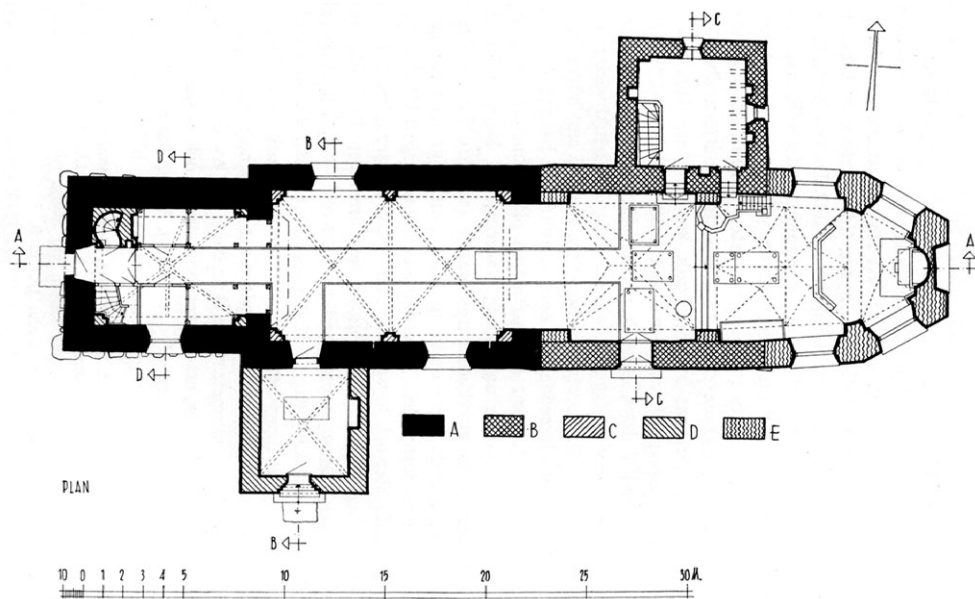
Plan av kyrkan mot norr. Uppmätning J Söderberg 1956. Ur Sveriges kyrkor.
