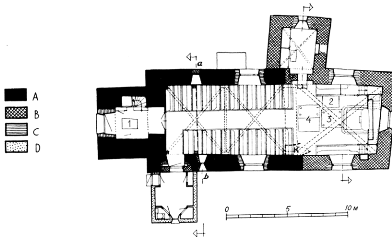
Plan av Eds kyrka mot norr. Uppmätning av R Bohlin och P Hedquist 1916, kompletterad av J Söderberg 1957. Sveriges kyrkor.
