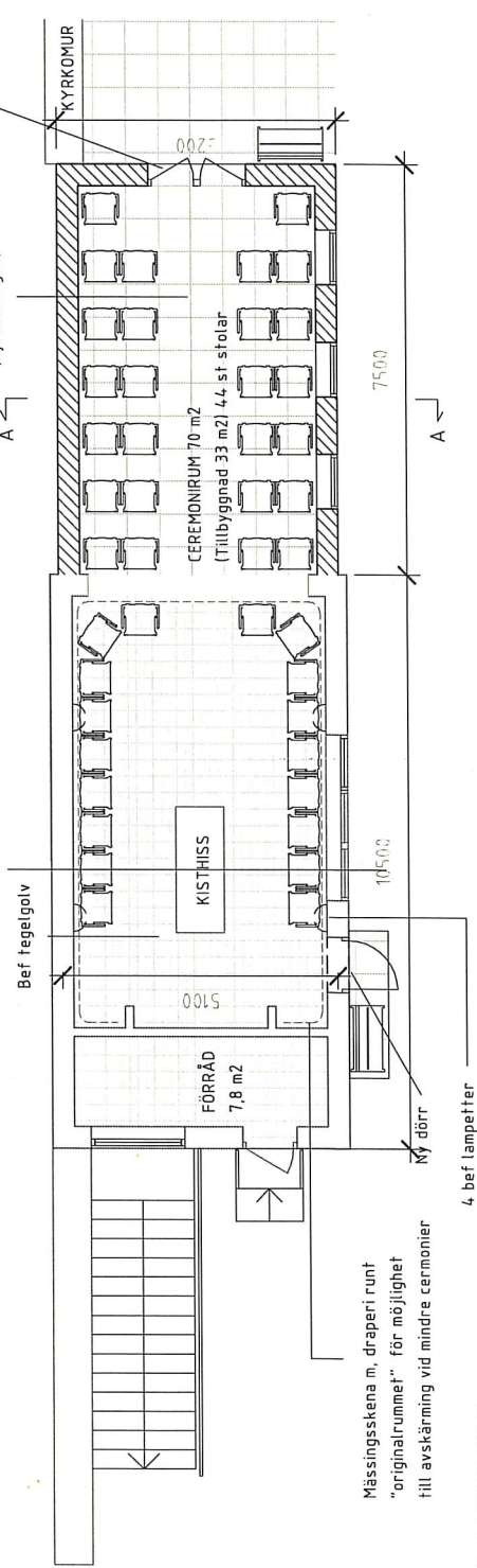
PLANRITNING
