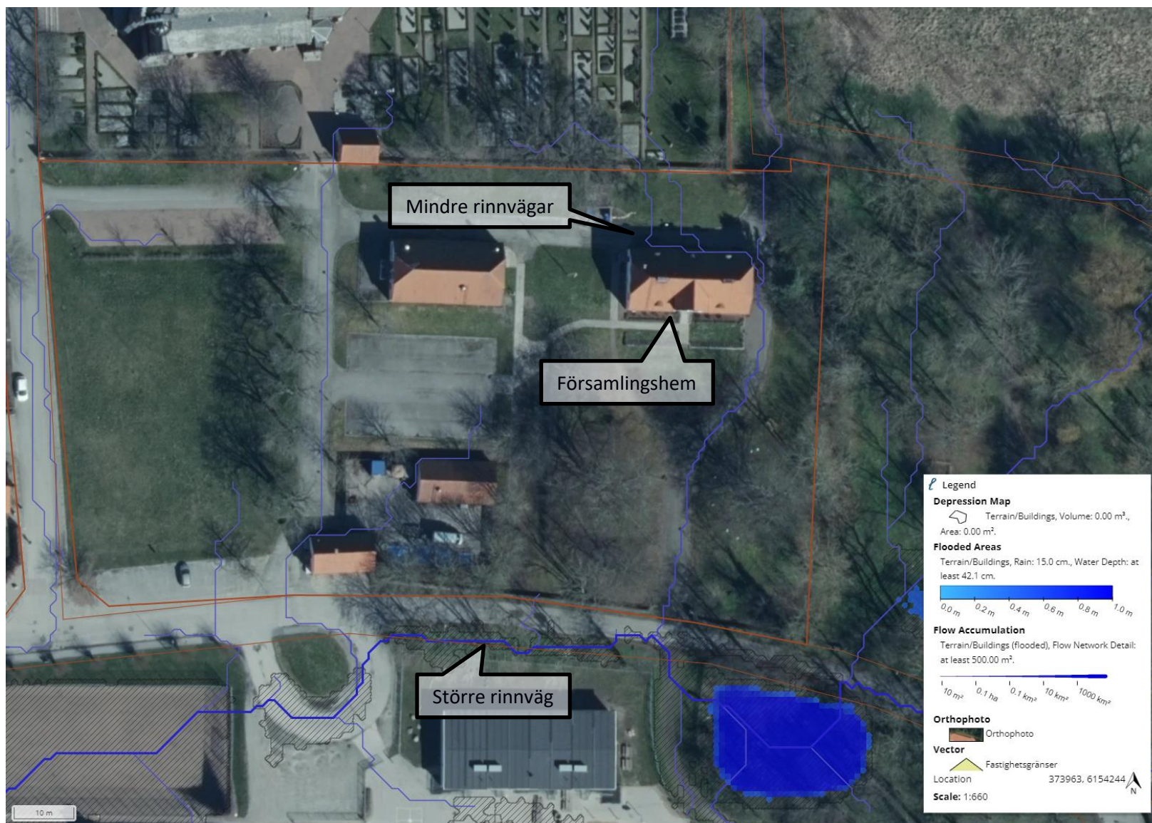
Figur 5. Översikt lågpunkter och rinnvägar, Tygelsjö och V. Klagstorps församlingshem
