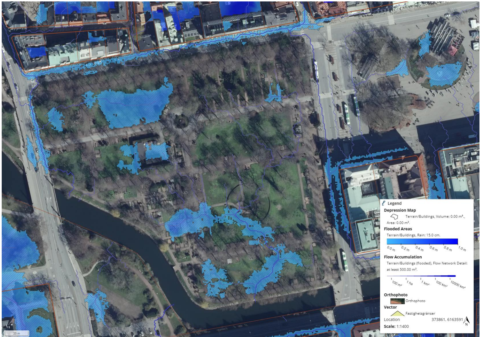
Översikt lågpunkter och rinnvägar, Gamla kyrkogården
