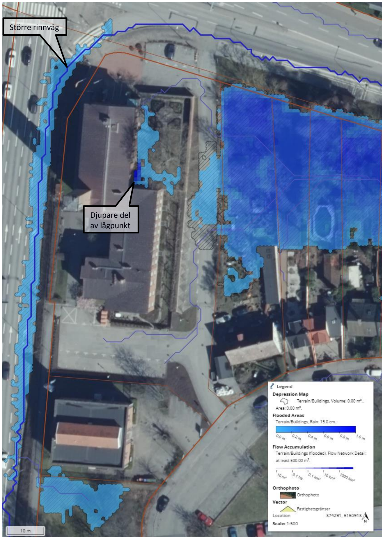
Figur 10. Översikt lågpunkter och rinnvägar, Heliga Trefaldighetskyrka.
