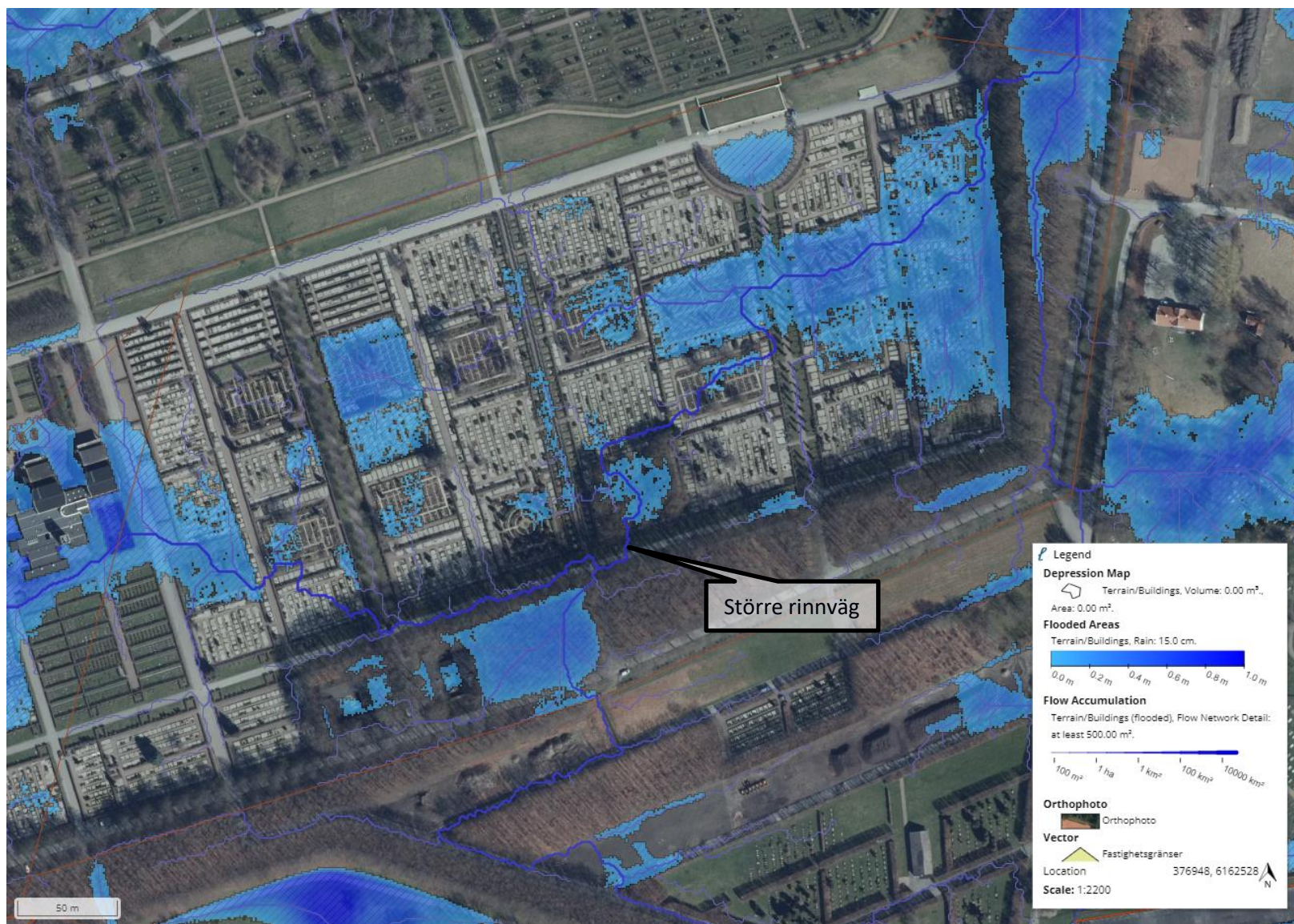
Figur 15. Översikt lågpunkter och rinnvägar Rosengård 170:3
