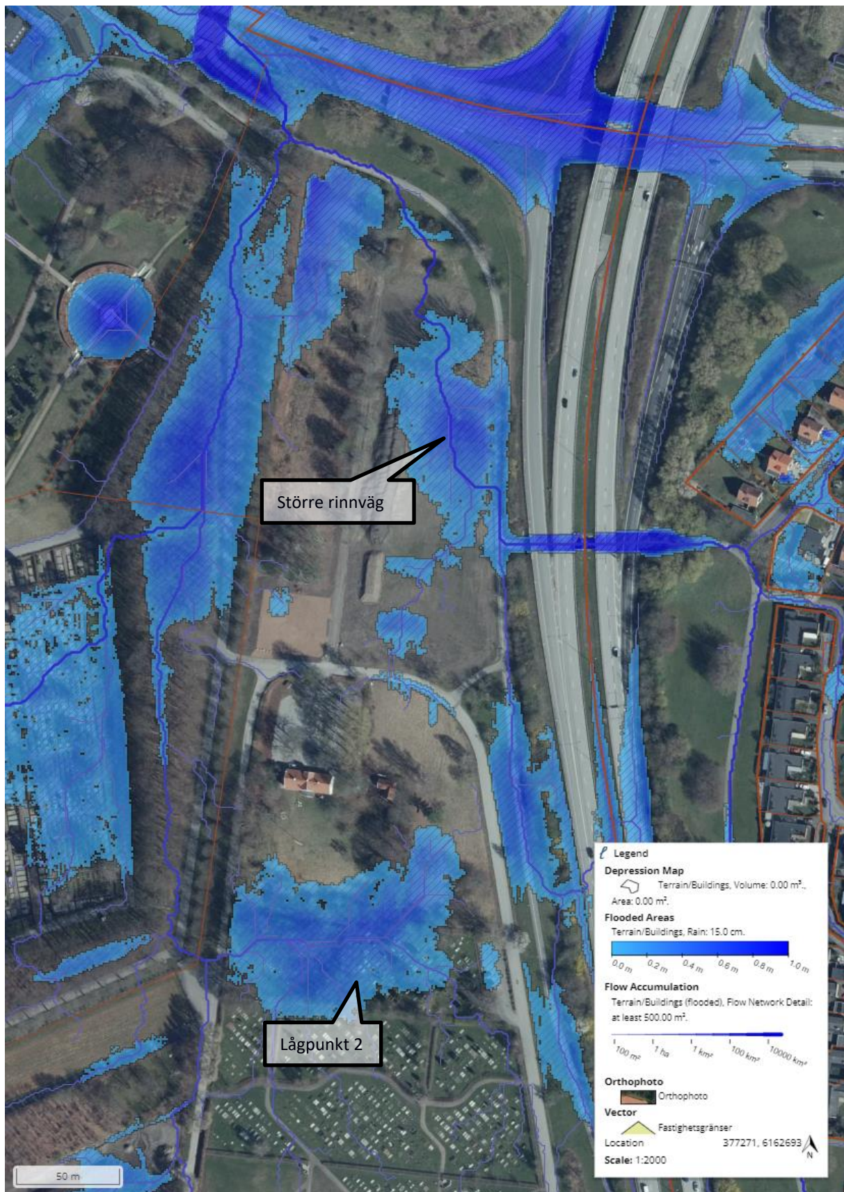
Figur 17. Översikt lågpunkter och rinnvägar, norra delen av Rosengård 170:4.
