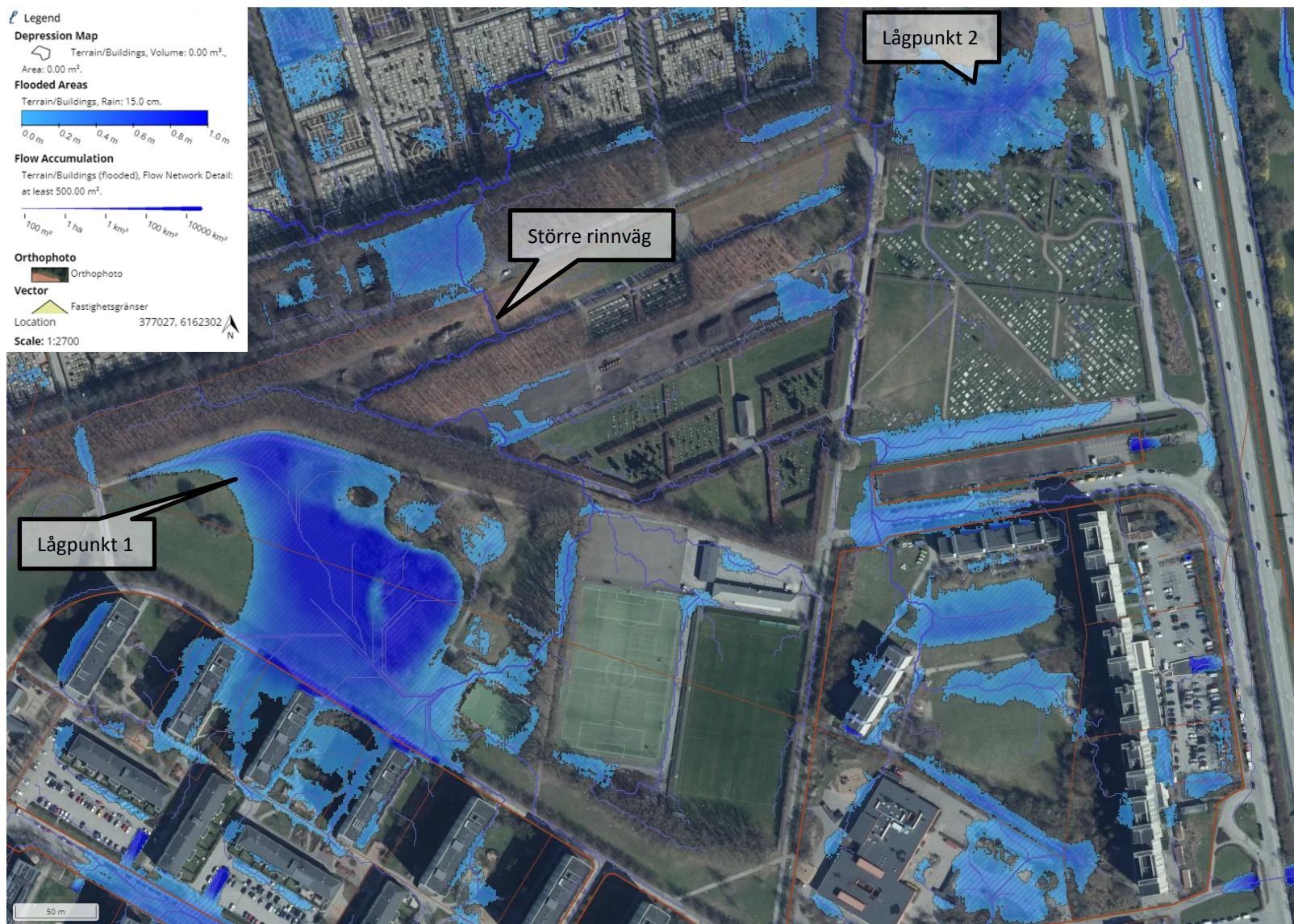
Figur 16. Översikt rinnvägar och lågpunkter, södra delen av Rosengård 170:4
