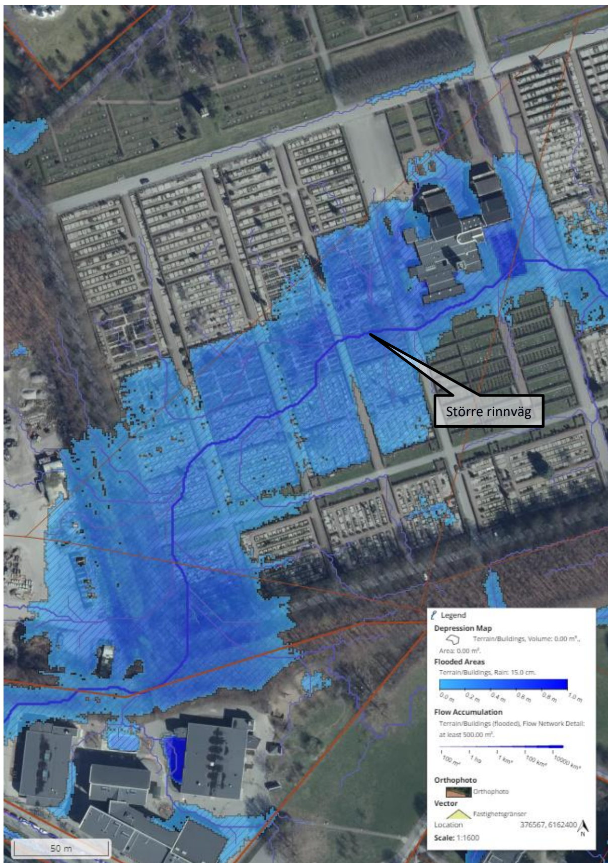
Figur 14. Översikt lågpunkter och rinnvägar, Rosengård 170:2
