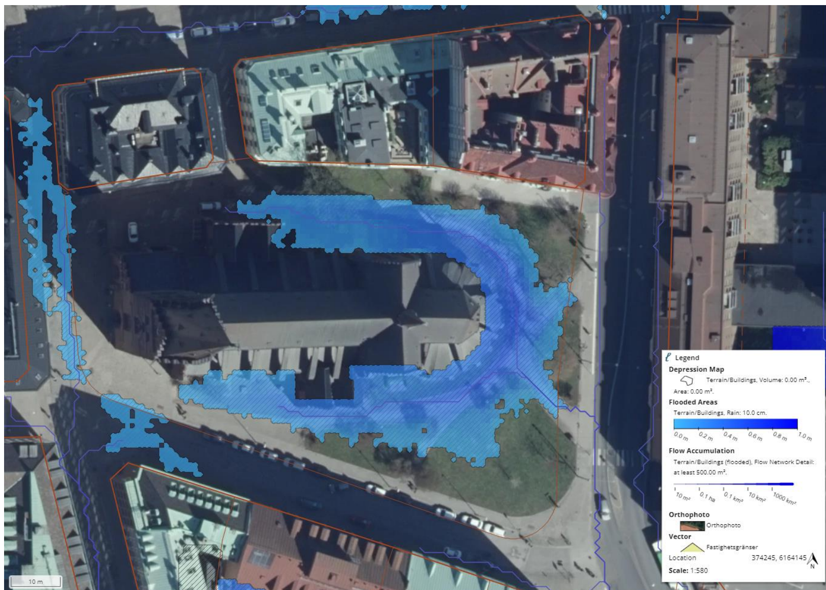
Figur 9. Översikt lågpunkter och rinnvägar, S:t Petri kyrka.
