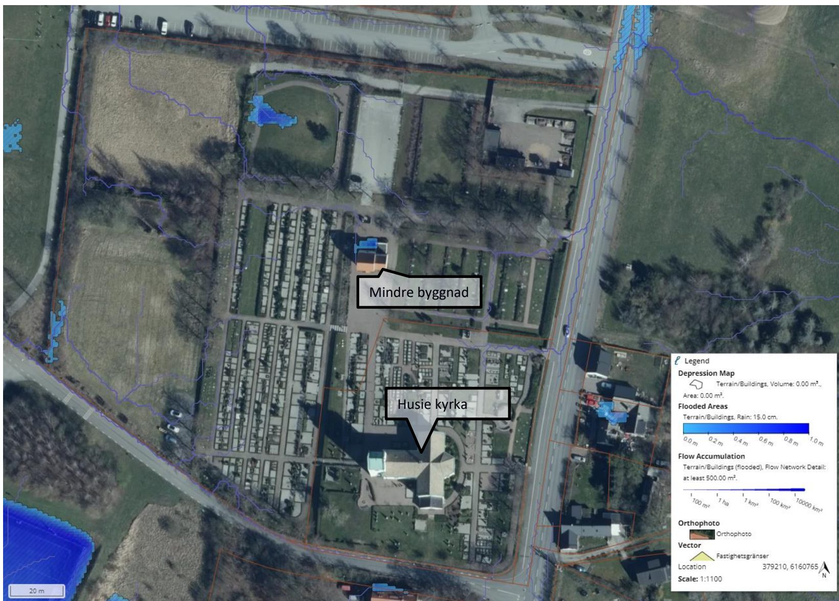
Figur 3. Översikt lågpunkter och rinnvägar, Husie kyrka och kyrkogård
