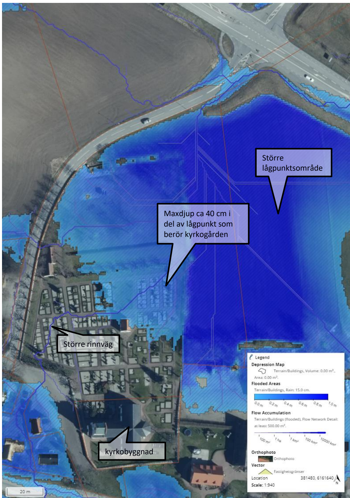
Figur 4. Översikt lågpunkter och rinnvägar Södra Sallerups kyrka.
