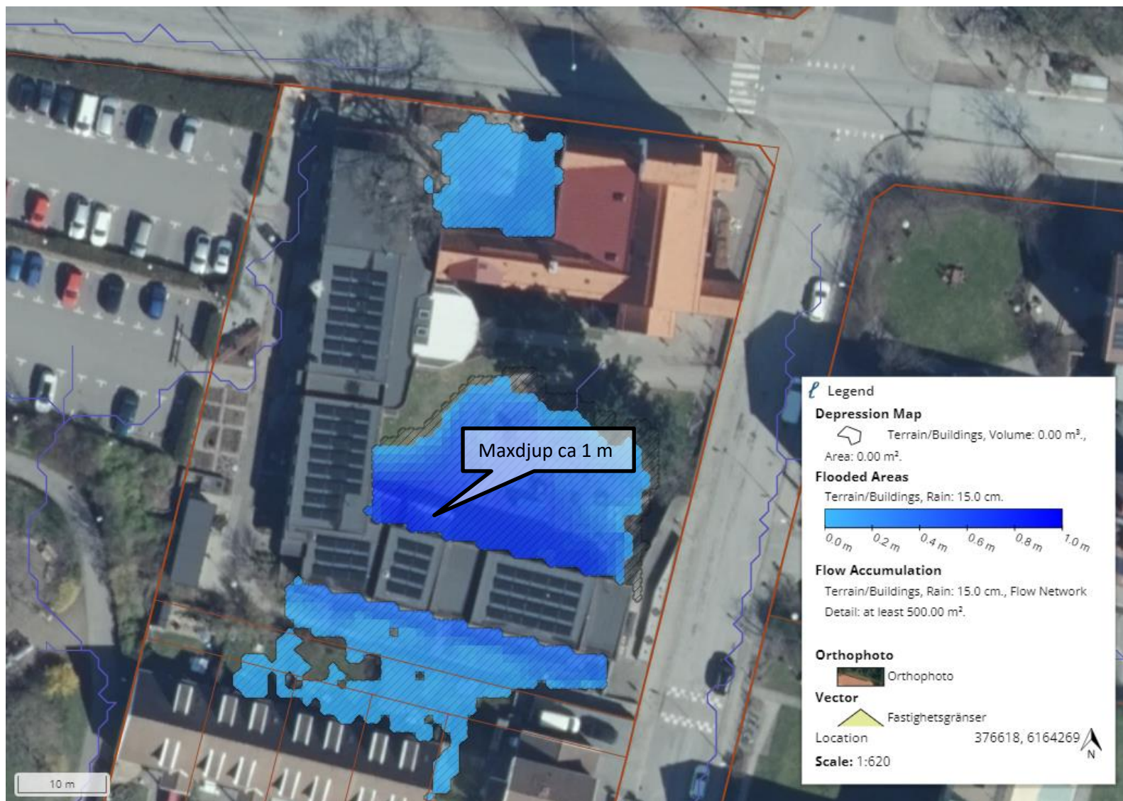
Figur 2. Översikt lågpunkter och rinnvägar Kirsebergs kyrka
