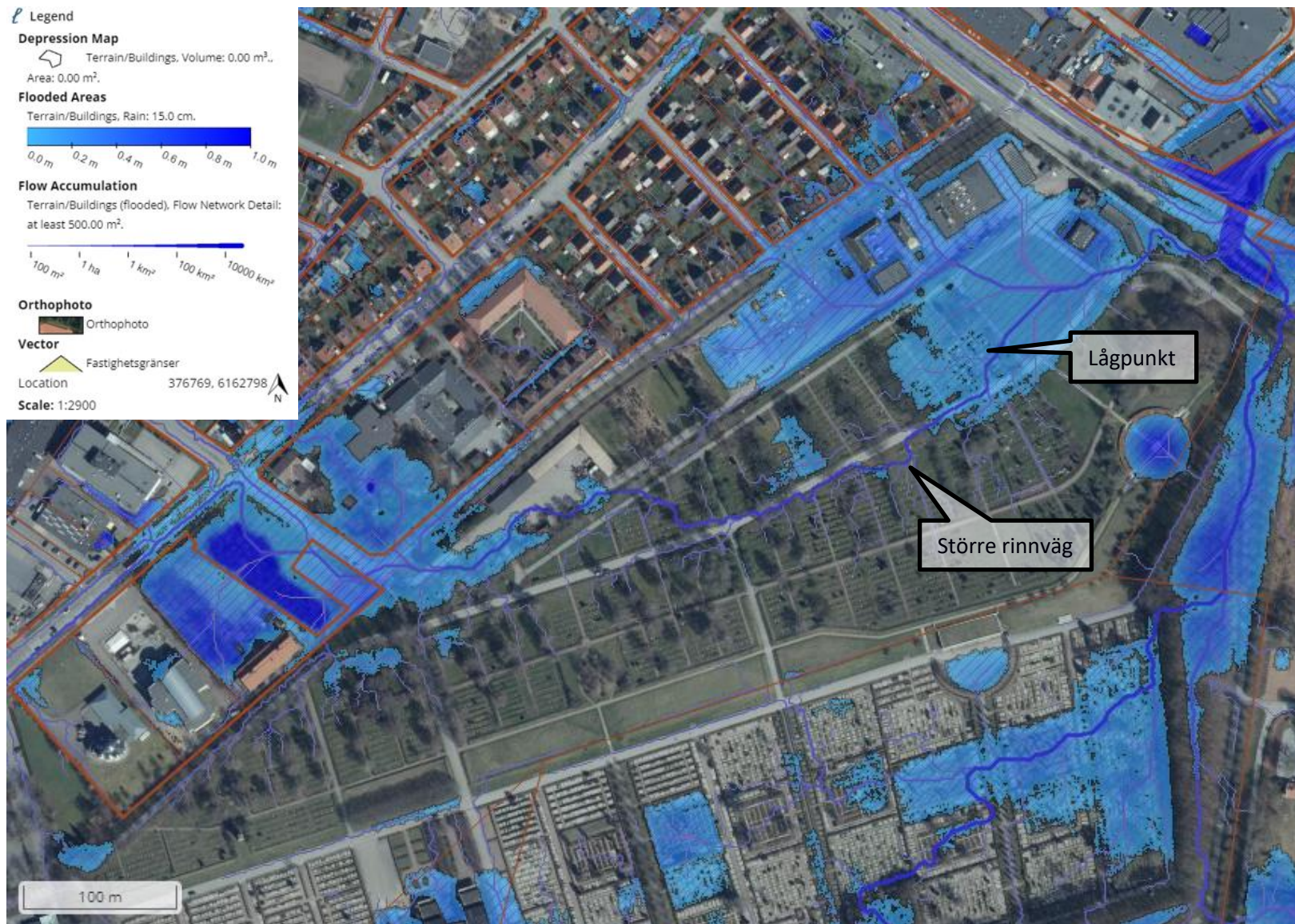
Figur 13. Översikt lågpunkter och rinnvägar, Rosengård 4:72.
