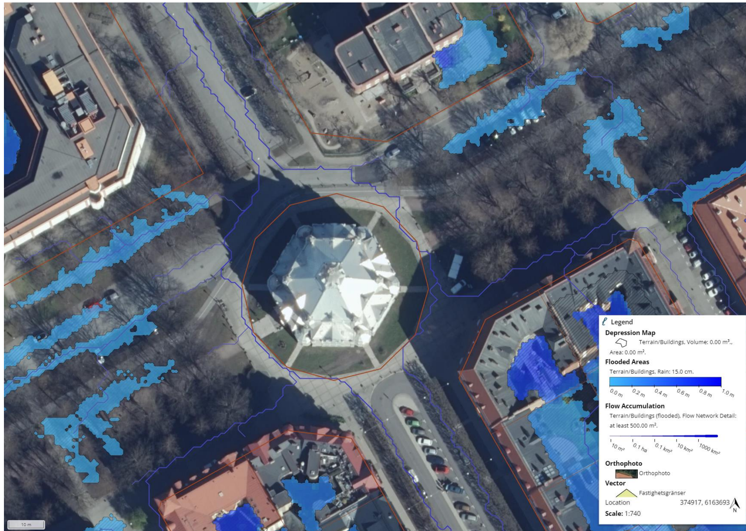
Figur 6. Översikt rinnvägar och lågpunkter, S:t Pauli kyrka.
