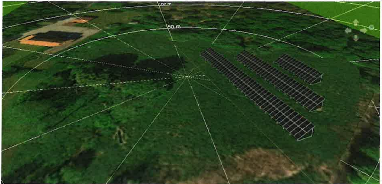
Illustration: 172st 550W paneler på markstativ till 80kW PRO växelriktare
