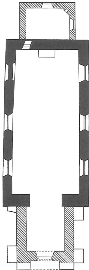
Åkerby kyrkas plan.
